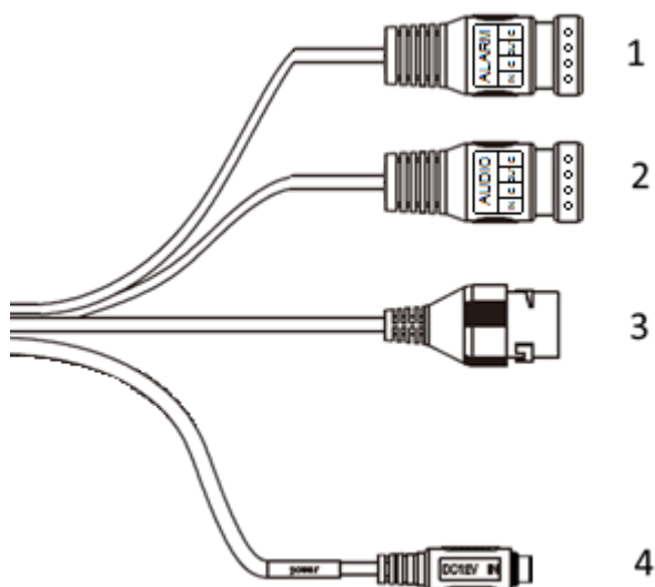
Рис. 2.1 Коммутационный кабель
